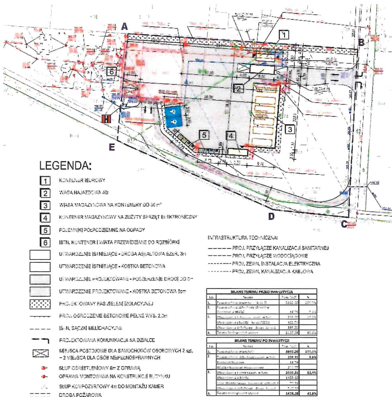
Schemat zagospodarowania przestrzennego projektowanego PSZOK w Zawadach.
